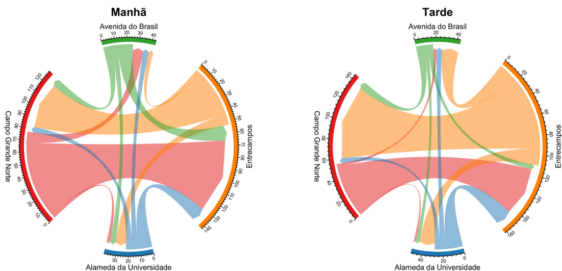
Figura 107: Fluxo direcional médio de ciclistas por hora no ponto B2 – Campo Grande / Alameda da Universidade / Av. do Brasil.
