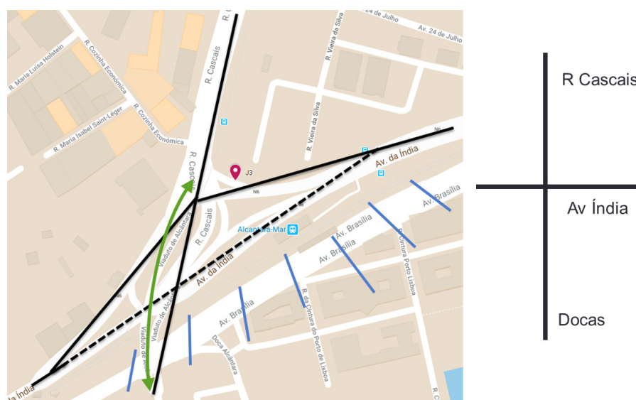
Figura 185: Simplificação do cruzamento J3 – Av. Índia / R Cascais / Viadutos. Nesta situação, não contar aqueles que passam na Av. Brasília, mas contar os que passam no viaduto.
