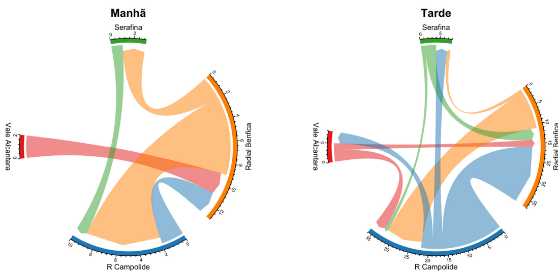
Figura 166: Fluxo direcional médio de ciclistas por hora no ponto N5 – Radial de Benfica / Rua de Campolide.
