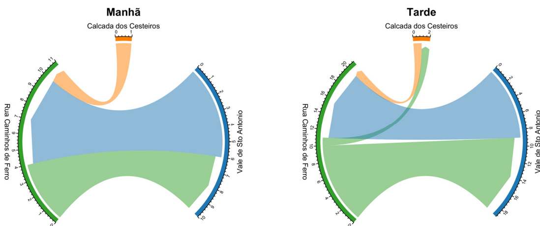
Figura 150: Fluxo direcional médio de ciclistas por hora no ponto J5 – R Caminhos de Ferro / Vale Santo António / Cç Cesteiros.
