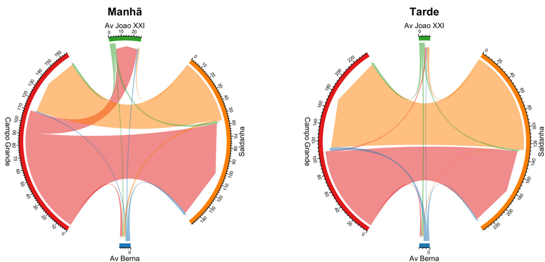
Figura 113: Fluxo direcional médio de ciclistas por hora no ponto C3 – Av. da República / Av. de Berna.
