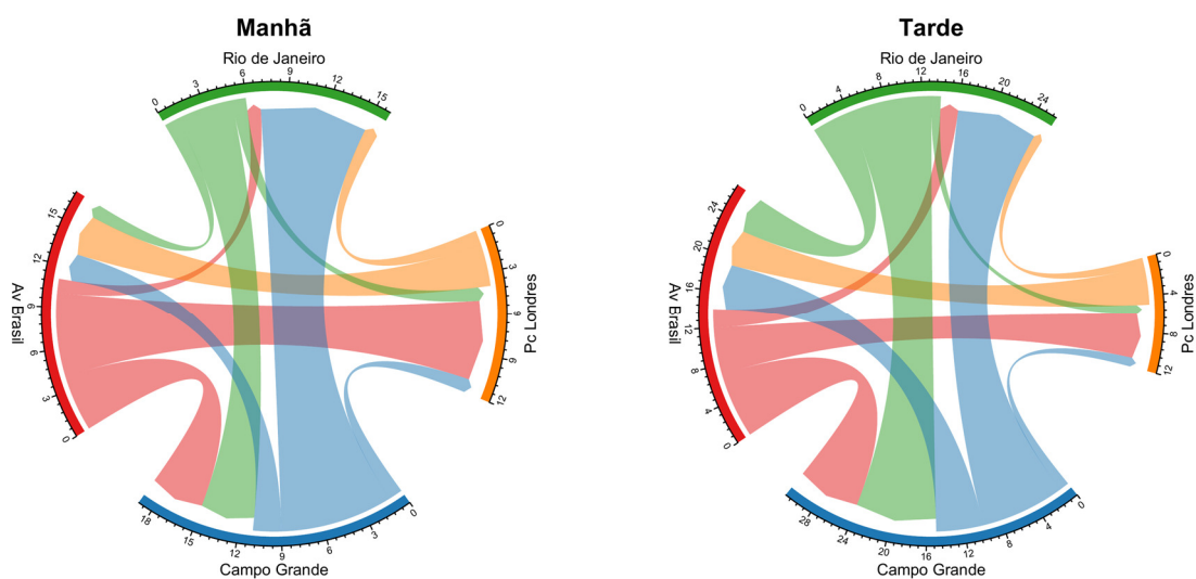
Figura 154: Fluxo direcional médio de ciclistas por hora no ponto L4 – Praça de Alvalade / Av. Roma / Av. Igreja.
