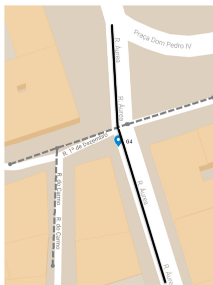
Figura 180: Simplificação do cruzamento G4 – Rua do Ouro / Rua do Carmo, Rossio.
