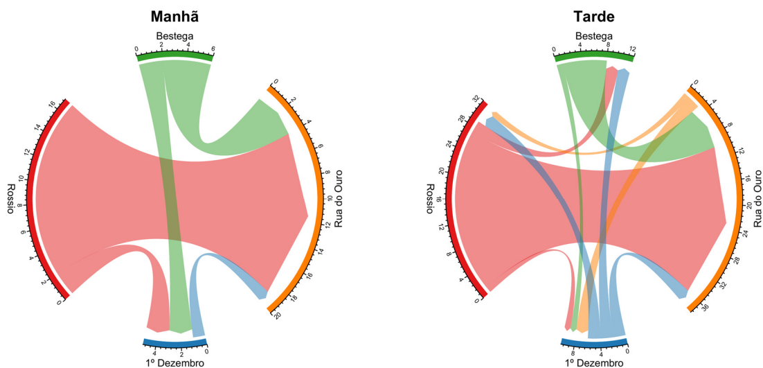
Figura 134: Fluxo direcional médio de ciclistas por hora no ponto G4 – Rua do Ouro / Rua do Carmo, Rossio.
