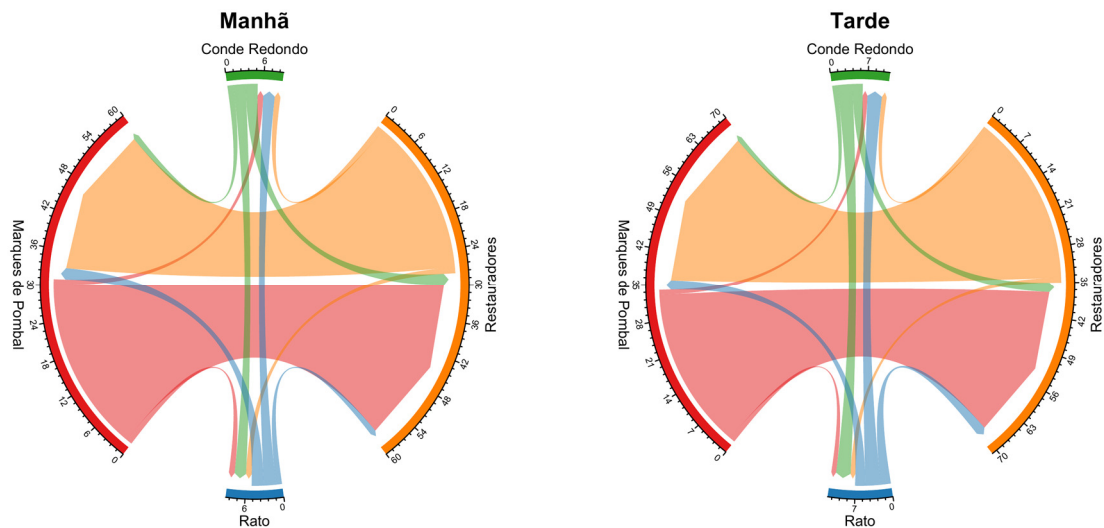
Figura 132: Fluxo direcional médio de ciclistas por hora no ponto G2 – Av. da Liberdade / Av. Alexandre Herculano.
