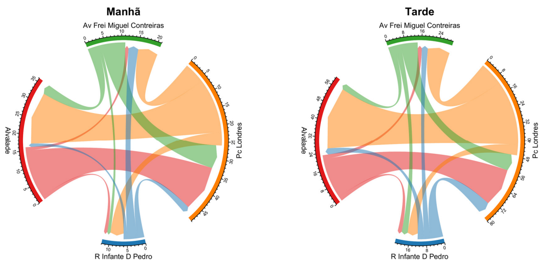
Figura 116: Fluxo direcional médio de ciclistas por hora no ponto D1 – Av. Roma / Av. Frei Miguel Contreiras.
