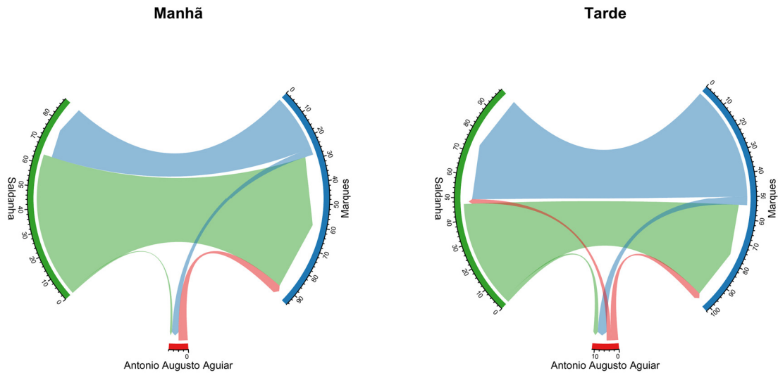
Figura 131: Fluxo direcional médio de ciclistas por hora no ponto G1 – Av. Fontes Pereira de Melo / Av. António Augusto Aguiar.
