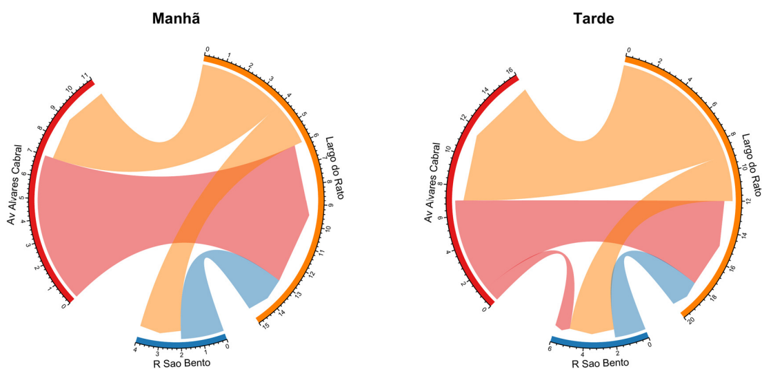
Figura 135: Fluxo direcional médio de ciclistas por hora no ponto G5 – Av. Álvares Cabral / R de São Bento / Largo do Rato.
