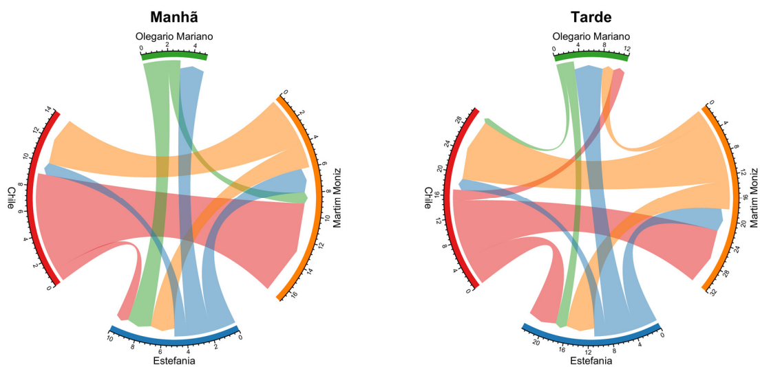
Figura 97: Fluxo direcional médio de ciclistas por hora no ponto H3 – Av. Almirante Reis / R Pascoal de Melo.
