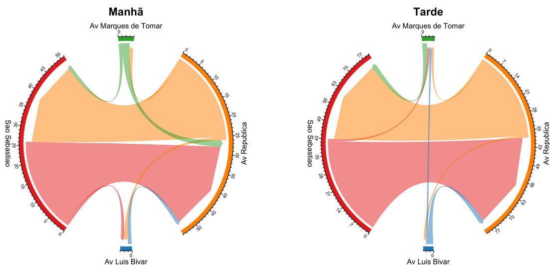
Figura 123: Fluxo direcional médio de ciclistas por hora no ponto E3 – Av. Duque d'Ávila / Luís Bívar, Marquês de Toma.
