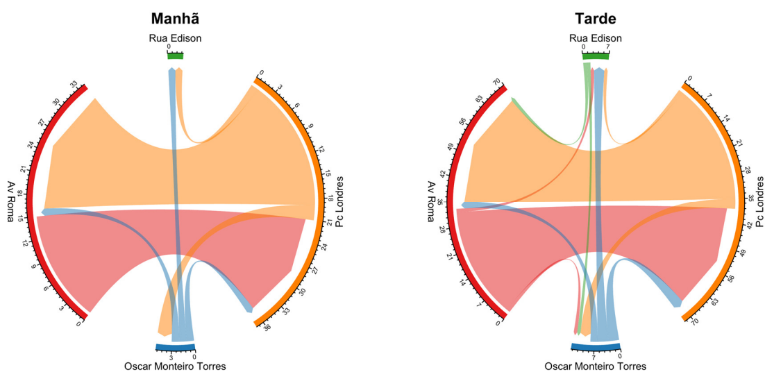
Figura 153: Fluxo direcional médio de ciclistas por hora no ponto L3 – Av. de Roma / Óscar Monteiro Torres / R Edison.
