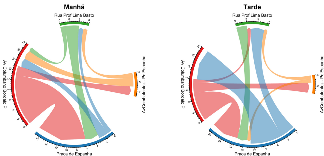
Figura 158: Fluxo direcional médio de ciclistas por hora no ponto M3 – Pç Espanha / Columbano Bordalo Pinheiro / Prof Lima Basto.
