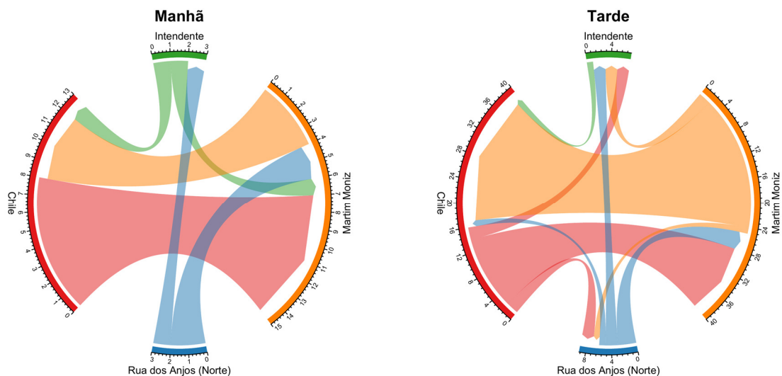
Figura 98: Fluxo direcional médio de ciclistas por hora no ponto H4 – Av. Almirante Reis / Rua dos Anjos.
