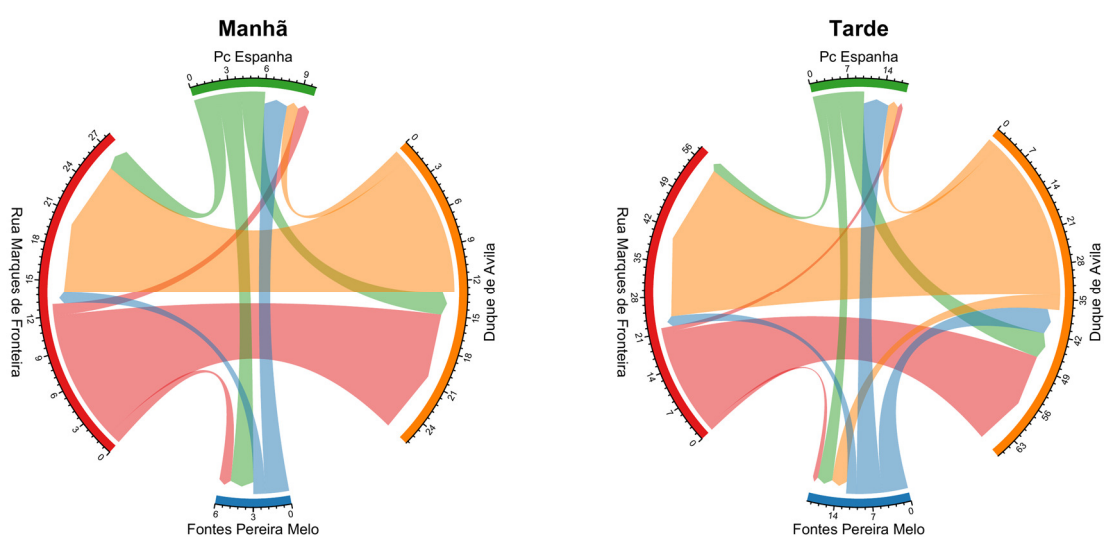
Figura 93: Fluxo direcional médio de ciclistas por hora no ponto E2 – R Marquês de Fronteira / Av. António Augusto Aguiar.
