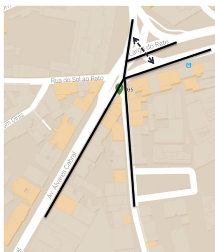
Figura 181: Simplificação do entroncamento G5 – Av. Álvares Cabral / R de São Bento / Largo do Rato.
