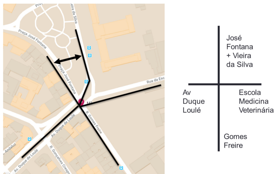
Figura 190: Simplificação do cruzamento M2 – Av. Duque de Loulé / R Gomes Freire / R Medicina Veterinária / Pç José Fontana.
