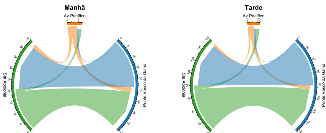
Figura 92: Fluxo direcional médio de ciclistas por hora no ponto D5 – Alameda dos Oceanos / Av. Pacífico.
