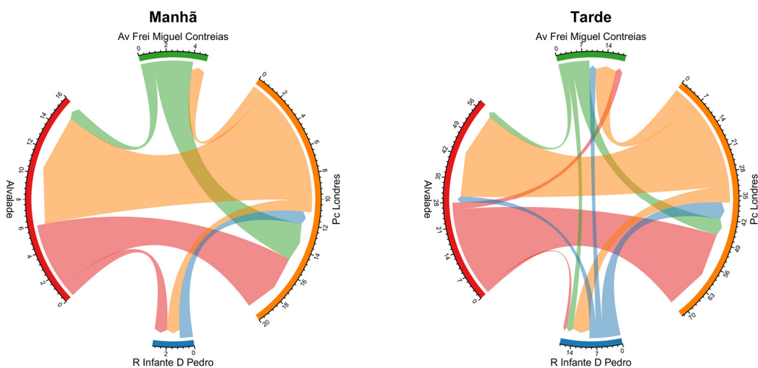
Figura 90: Fluxo direcional médio de ciclistas por hora no ponto D1 – Av. de Roma / Av. Frei Miguel Contreiras.
