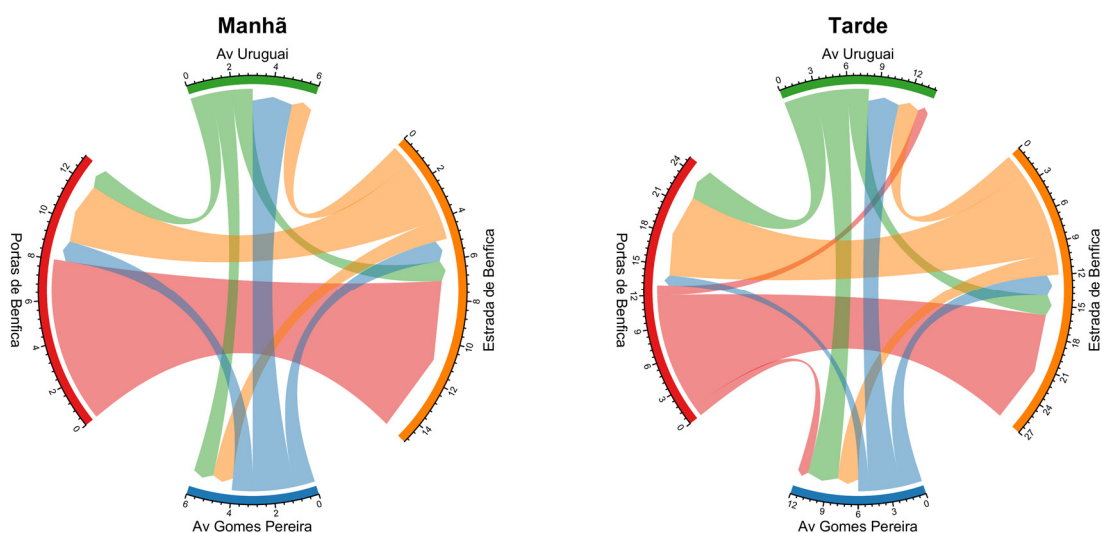
Figura 87: Fluxo direcional médio de ciclistas por hora no ponto A5 - Estrada de Benfica / Av. Uruguai / Av. Gomes Pereira.
