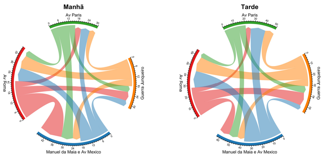
Figura 119: Fluxo direcional médio de ciclistas por hora no ponto D4 – Praça de Londres, Av. Guerra Junqueiro / Manuel da Maia / Av. Paris.
