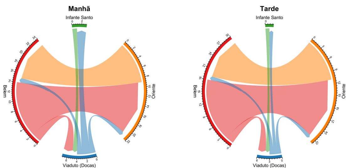
Figura 145: Fluxo direcional médio de ciclistas por hora no ponto I5 – Av. 24 de Julho / Av. Infante Santo.
