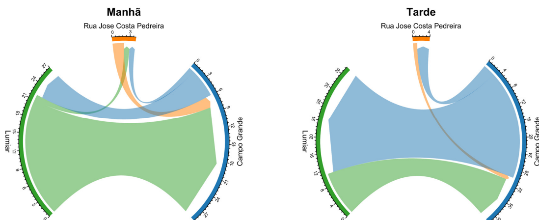
Figura 102: Fluxo direcional médio de ciclistas por hora no ponto A2 – Alameda das Linhas de Torres / R. José Costa Pedreira.
