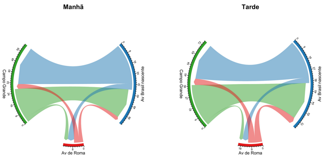
Figura 108: Fluxo direcional médio de ciclistas por hora no ponto B3 – Av. do Brasil / Av. de Roma.
