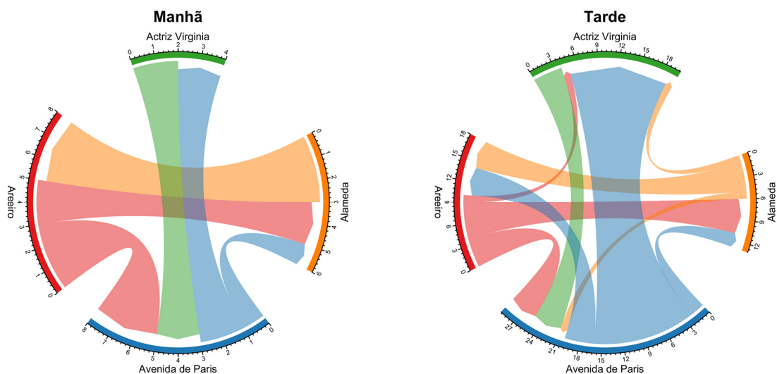
Figura 152: Fluxo direcional médio de ciclistas por hora no pontol2 – Av. Almirante Reis / Av. de Paris.
