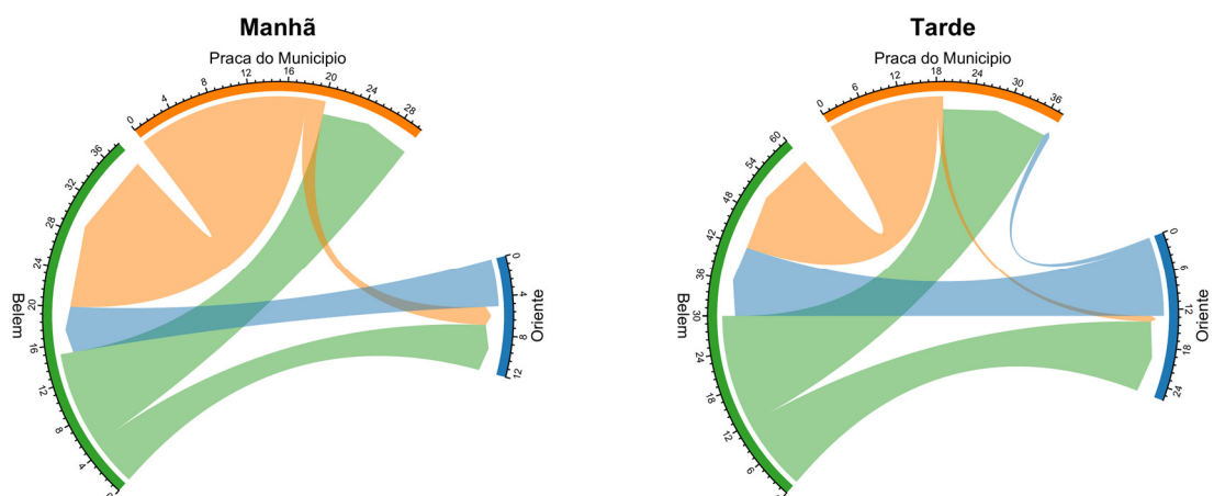
Figura 142: Fluxo direcional médio de ciclistas por hora no ponto I2 – Rua do Arsenal / Praça do Município.
