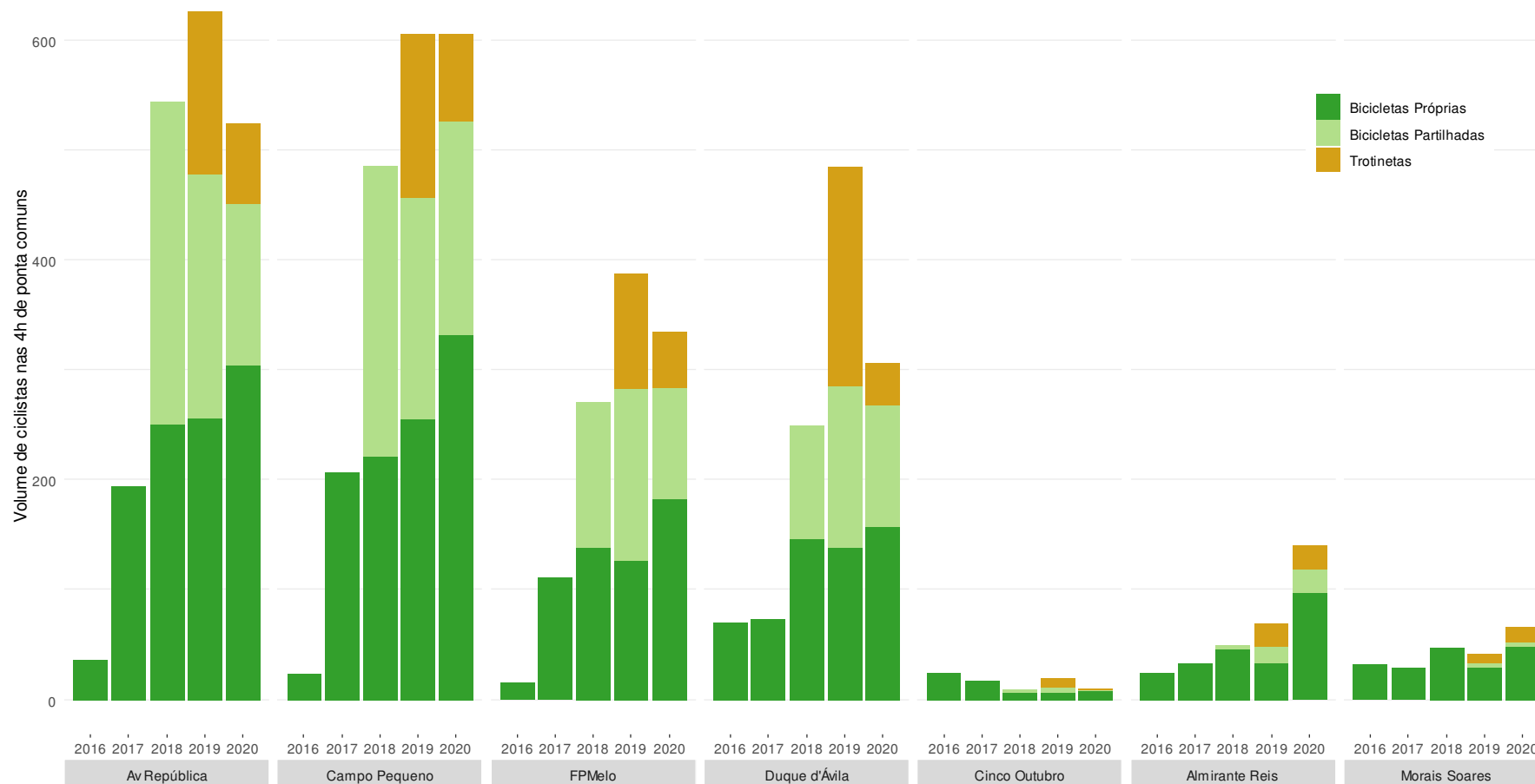
Figura 79: Comparação do volume de bicicletas e trotinetas observados em 7 locais em 2016 a 2020, durante as 4 horas de ponta observadas comparáveis.
