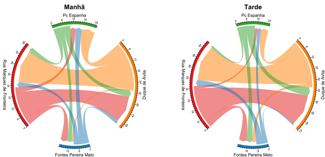
Figura 122: Fluxo direcional médio de ciclistas por hora no ponto E2 – Rua Marquês de Fronteira / Av. António Augusto Aguiar.
