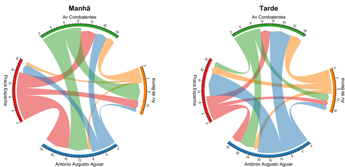
Figura 121: Fluxo direcional médio de ciclistas por hora no ponto E1 – Pç Espanha, Av. Berna / Av. António Augusto Aguiar.
