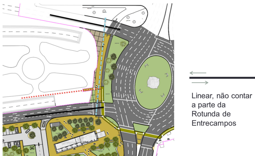
Figura 173: Simplificação do ponto C1 – Campo Grande, final da ciclovia (Entrecampos).
