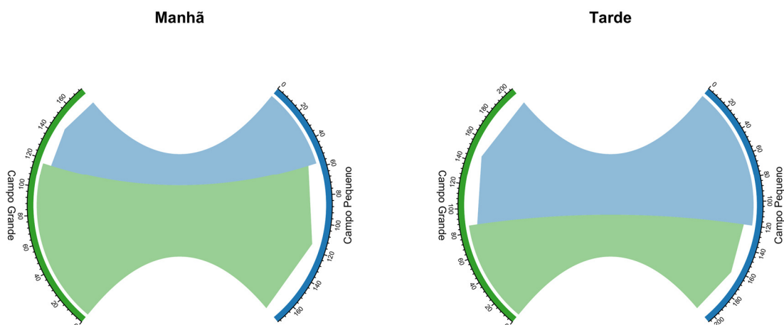
Figura 112: Fluxo direcional médio de ciclistas por hora no ponto C2 – Entrecampos, antes do viaduto comboios.
