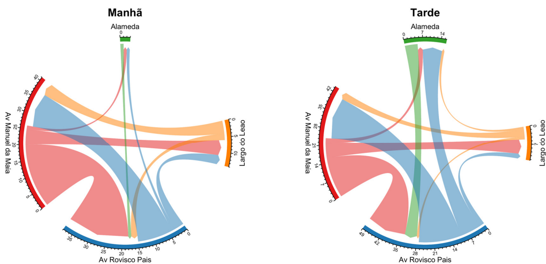
Figura 136: Fluxo direcional médio de ciclistas por hora no ponto H1 – Av. Manuel da Maia / Av. Rovisco Pais / Alameda.
