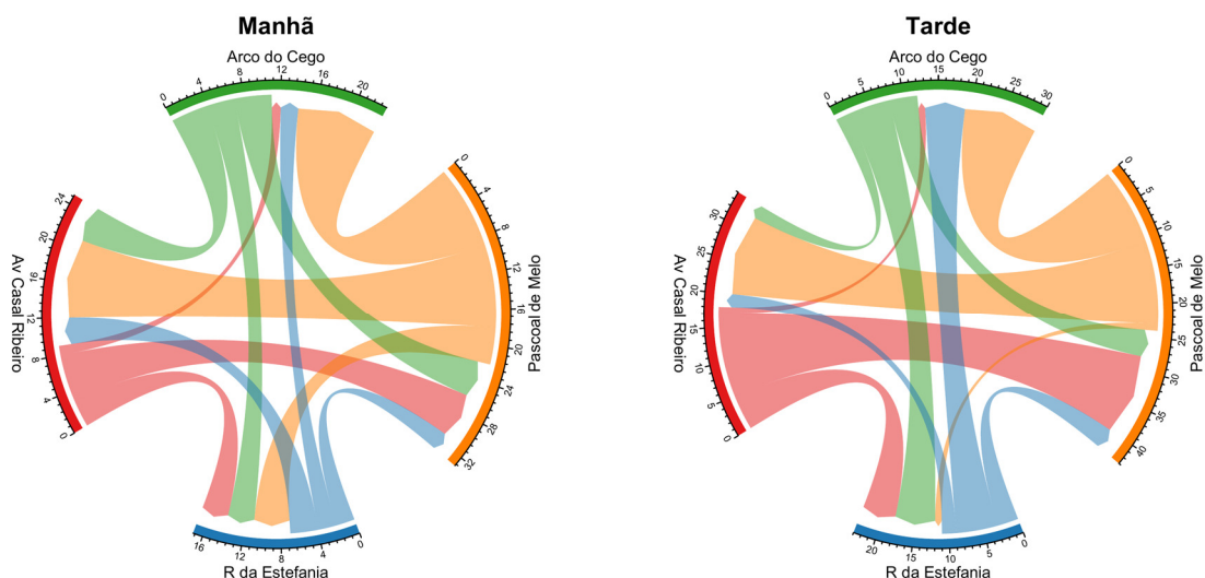
Figura 128: Fluxo direcional médio de ciclistas por hora no ponto F3 – Estefânia, R D Estefânia / Pascoal de Melo / Av. Casal Ribeiro.
