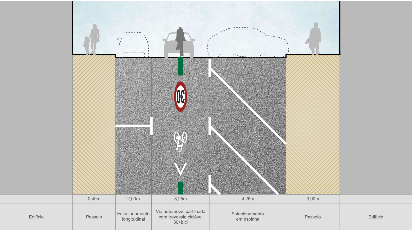
PERFIL TIPO - SITUAÇÃO PROPOSTA Rua Azado Gneco escala 1:100 Nota: As dimensões indicadas foram seleccionadas como representativas da globalidade do projeto
