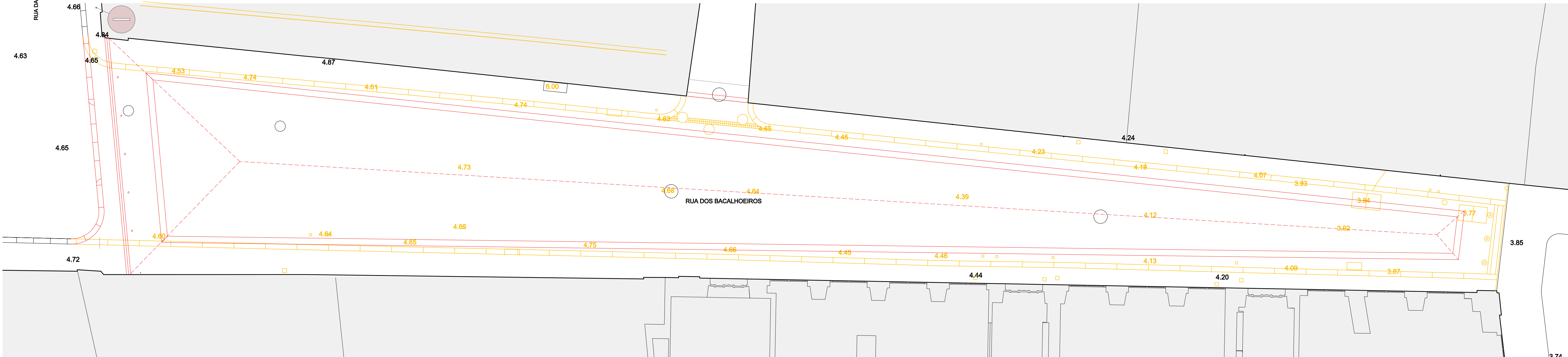
3 PLANTA DE ALTERAÇÕES PLANTA PARCIAL DA RUA DOS BACALHOEIOS
