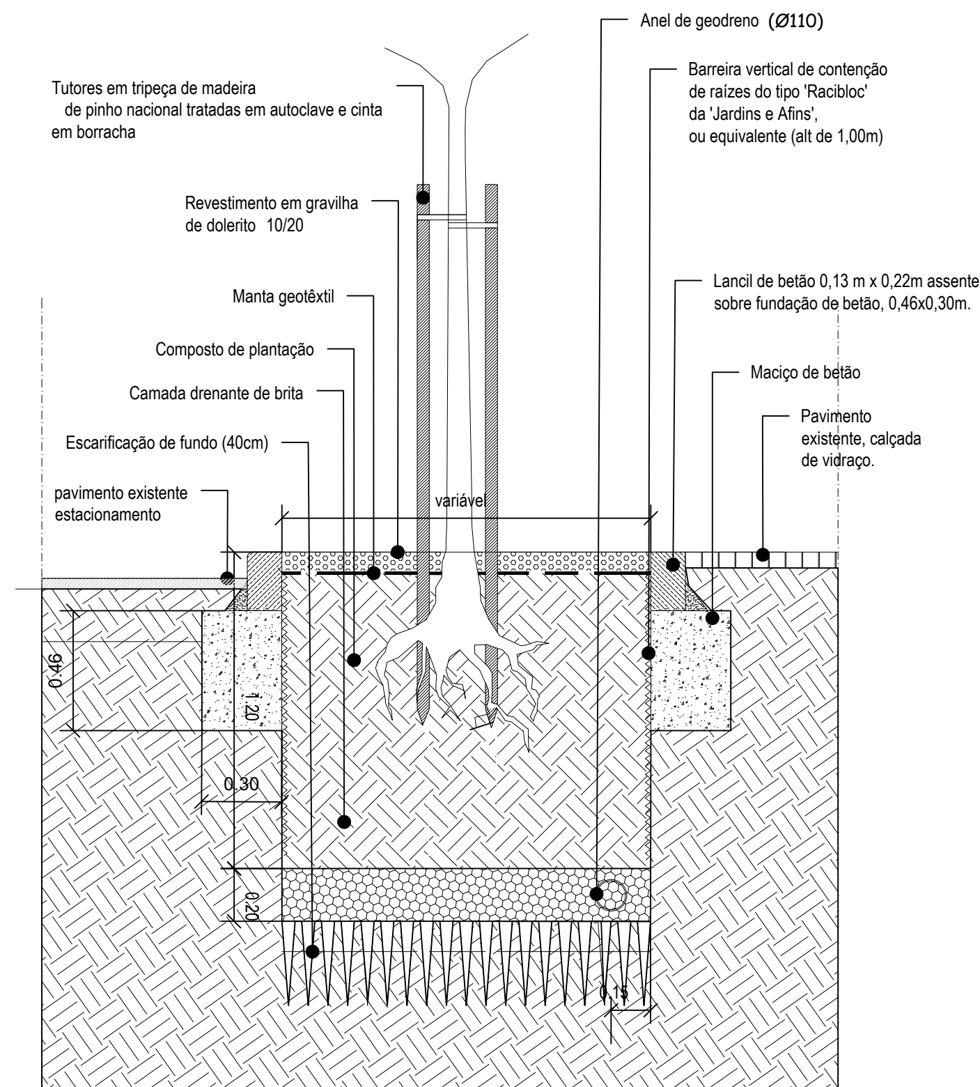
P1 Corte tipo de caldeira de árvore esc 1/20
