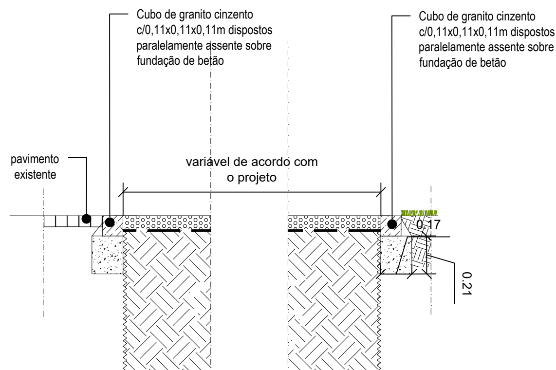
P3 Corte caldeira de árvore / cubo de granito. Ver também P1. (esc. 1/20)
