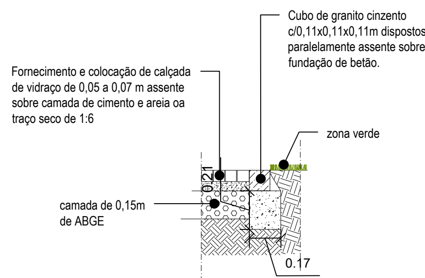
P4 Corte zona verde / calçada de vidro. (esc. 1/20)
