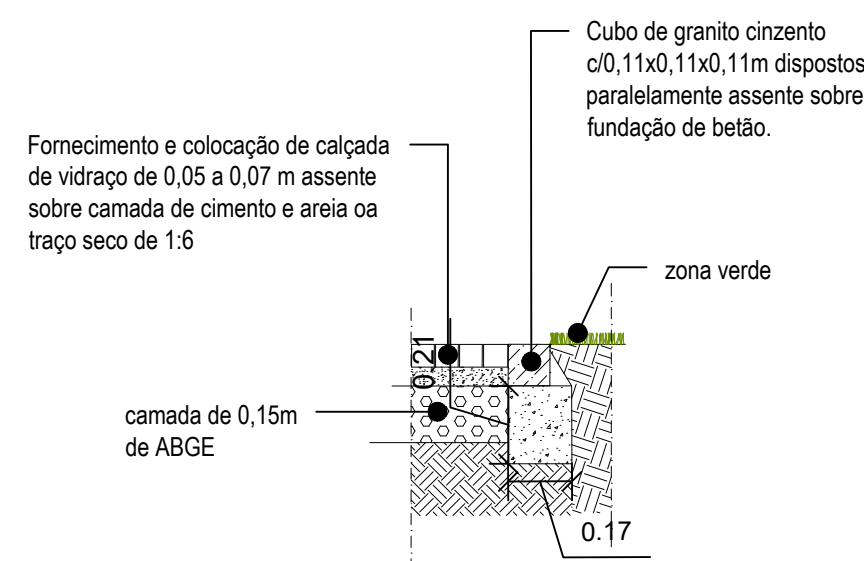
P4 Corte zona verde / calçada de vidroço. (esc. 1/20)
