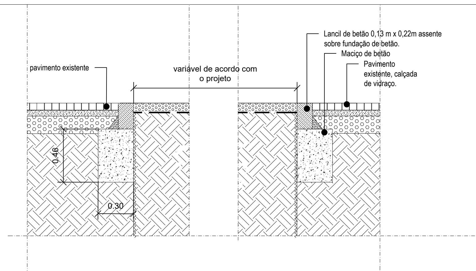
P2 Corte caldeira de árvore / lancil. Ver também o P1 - esc. 1/20
